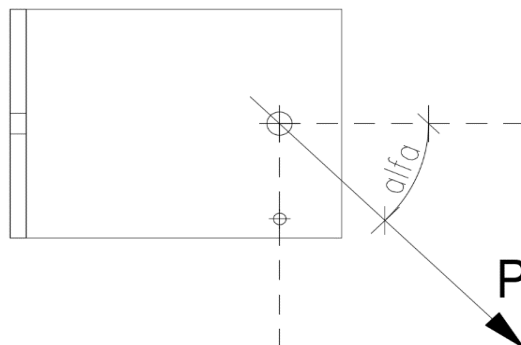
Rys. Dopuszczalne obciążenie na konsolę – schemat przyłożenia siły w zależności od kąta
